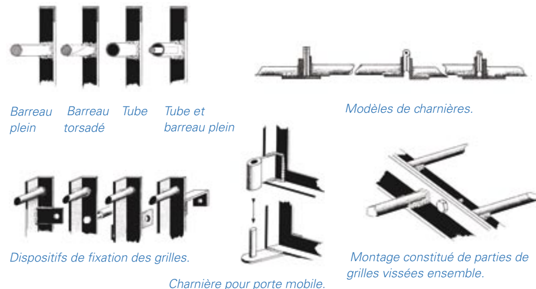
Figure 4. Détails de la fabrication des grilles.
