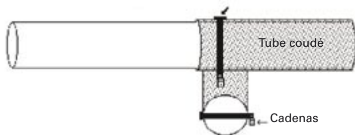
Figure 2. Grille utilisée en France. Les tubes d'acier, remplis de béton, cailloux et fers à béton, résistent à la découpe à la scie circulaire.
