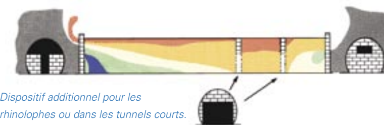
Site optimal offrant une gamme relativement stable de températures et humidités relatives. La dimension des dispositifs de fermeture dépend de la longueur du tunnel.
